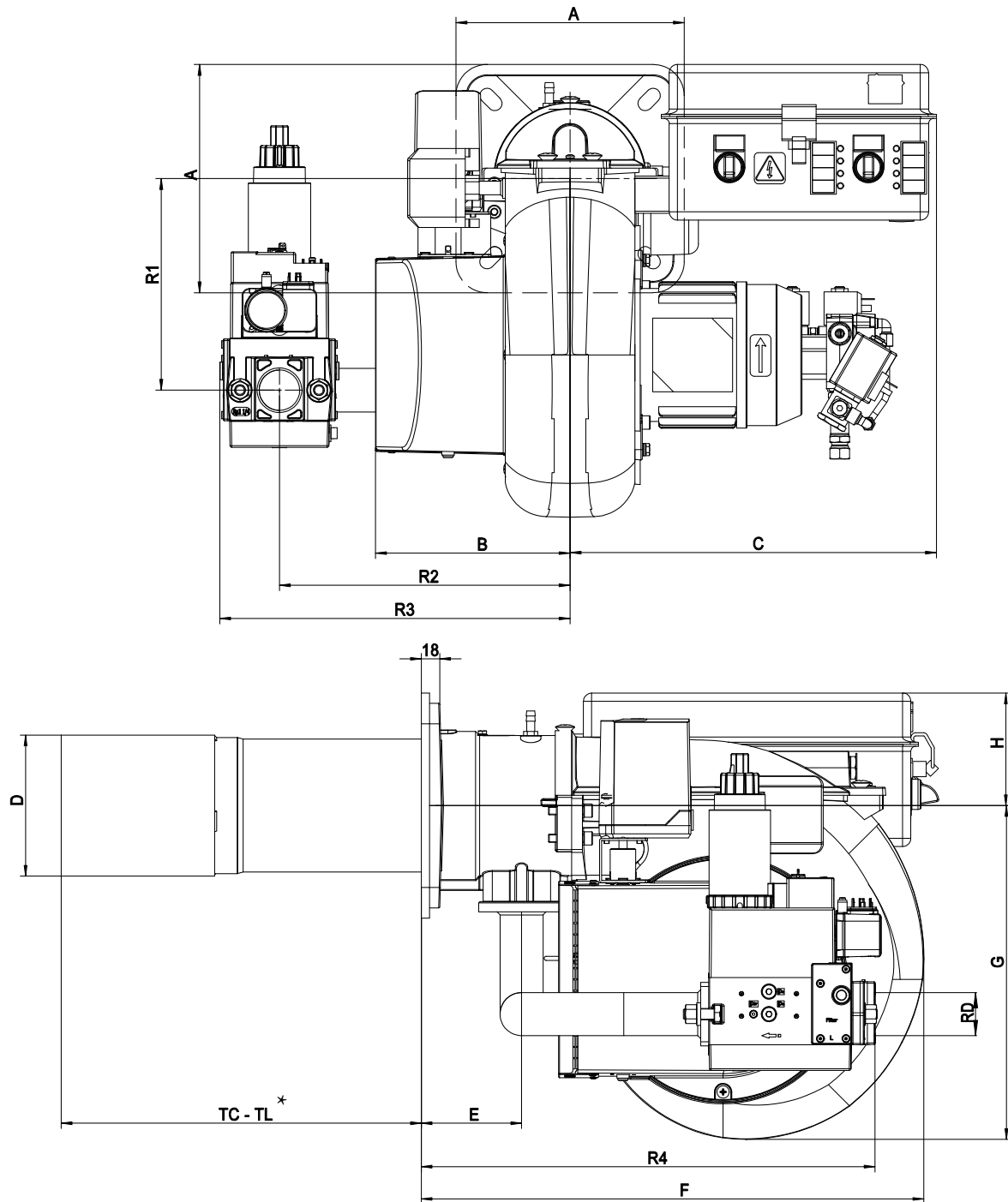
Fig. 3 Medidas K 3/2 - K 4/2
