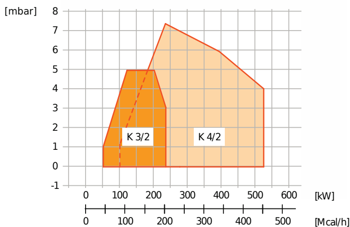
Fig. 2 X = Potencia térmica Y = Presión en la cámara de combustión
