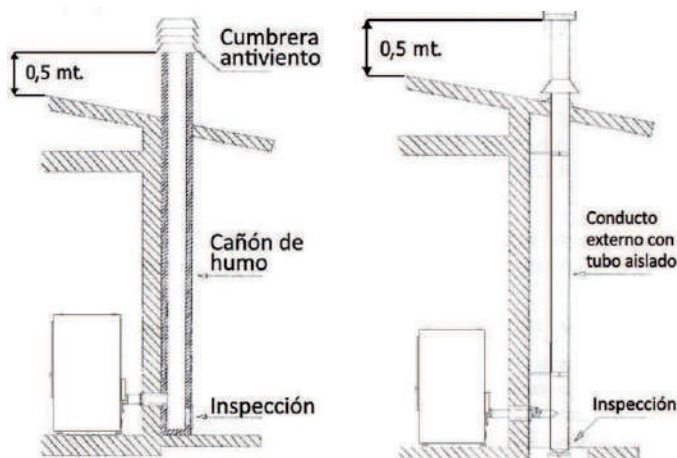
Fig. 3 : conexión a un conducto exterior con tubo aislado o doble pared una cumbrera antiviento.
