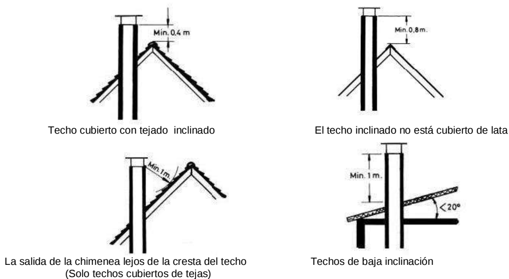
Figure 5 - Los tipos de montaje de la chimenea
