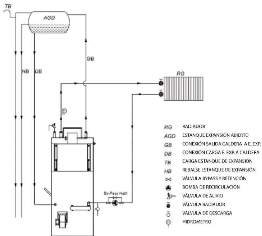
Figura 3 - Plano de instalación EKO B-20...-80
